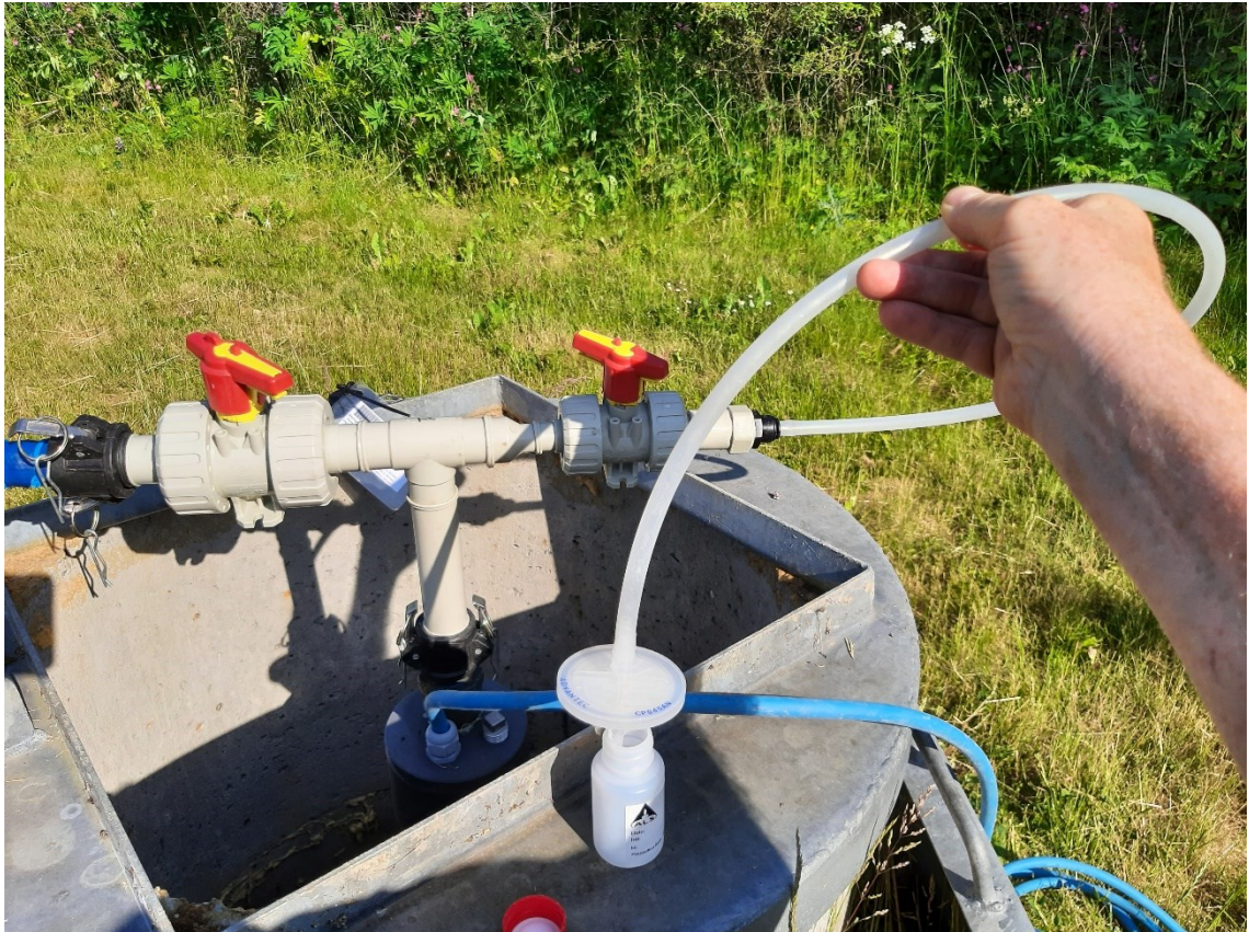
Figur 2. Online filtrering gennem engangsfilter ved hjælp af pumpetryk.
